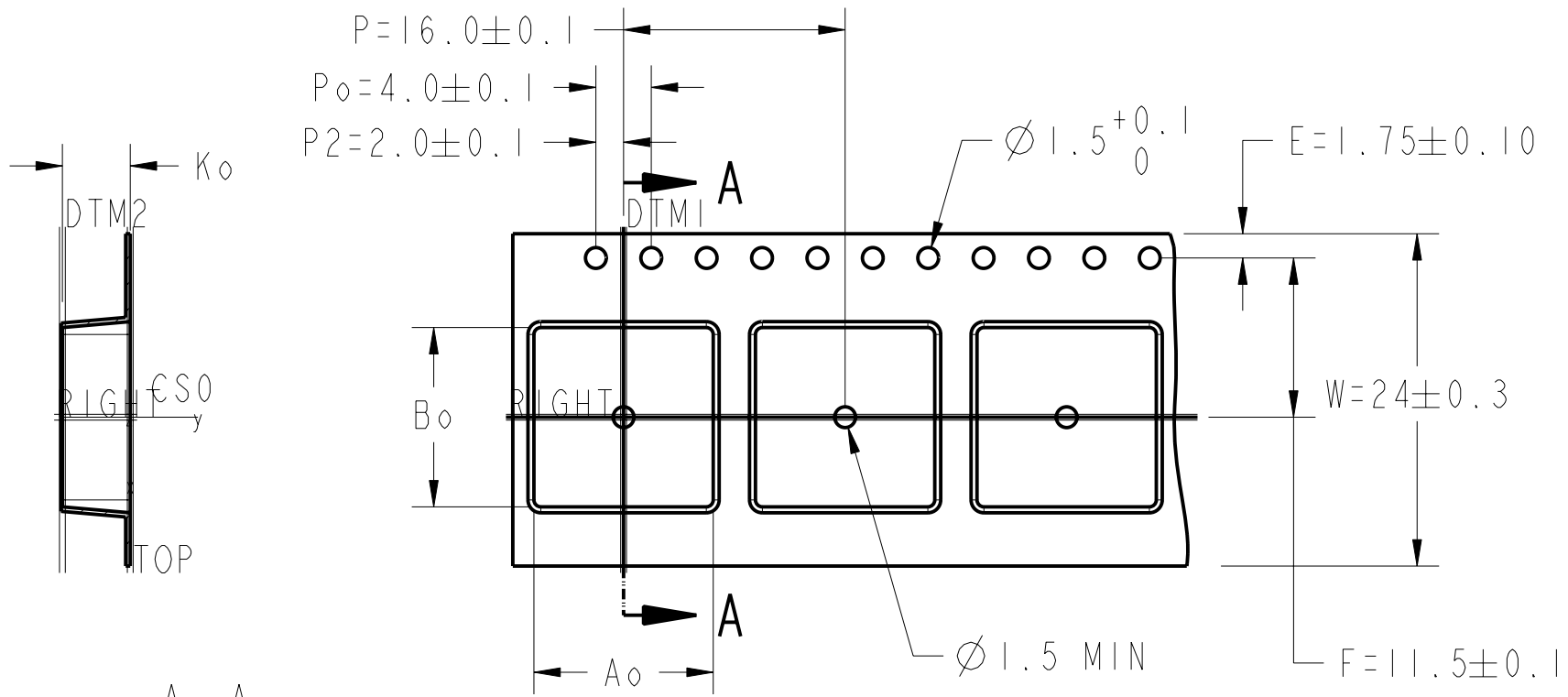
SECTION A-A
